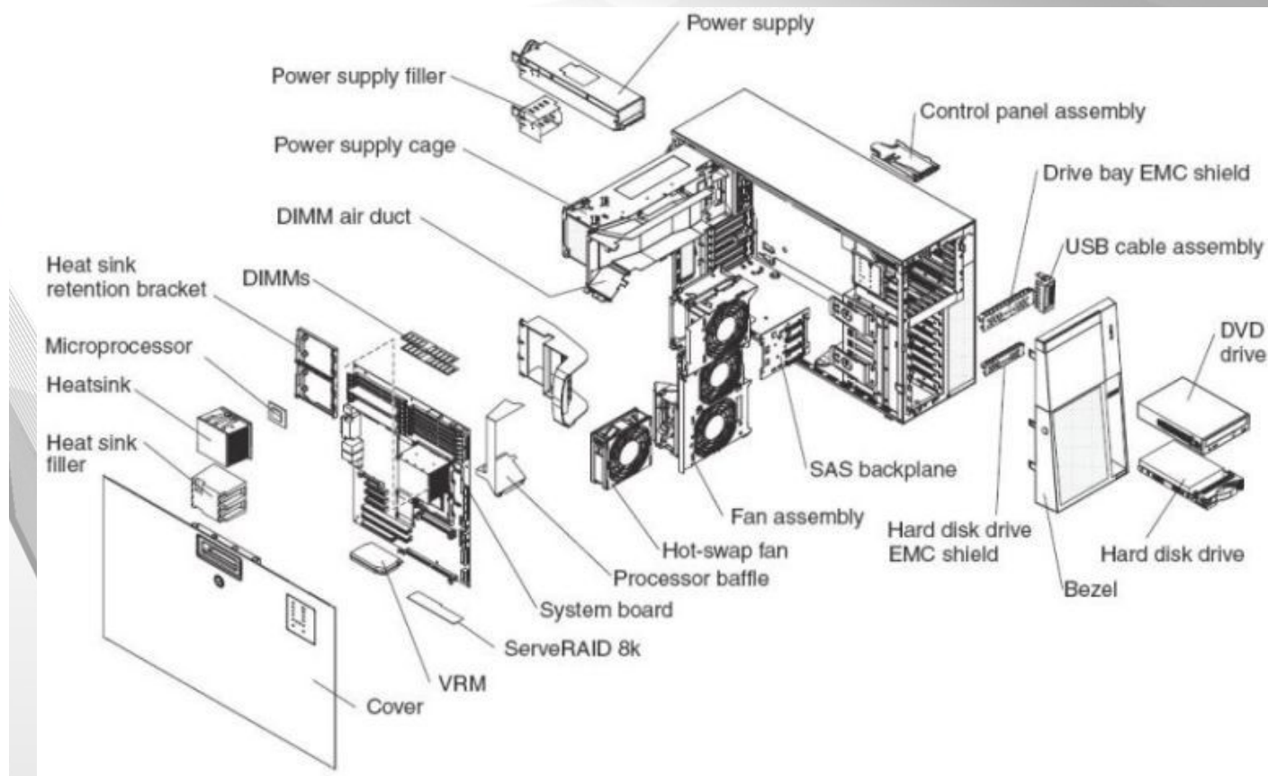
Рисунок 5 - Сервер IBM System x3500
