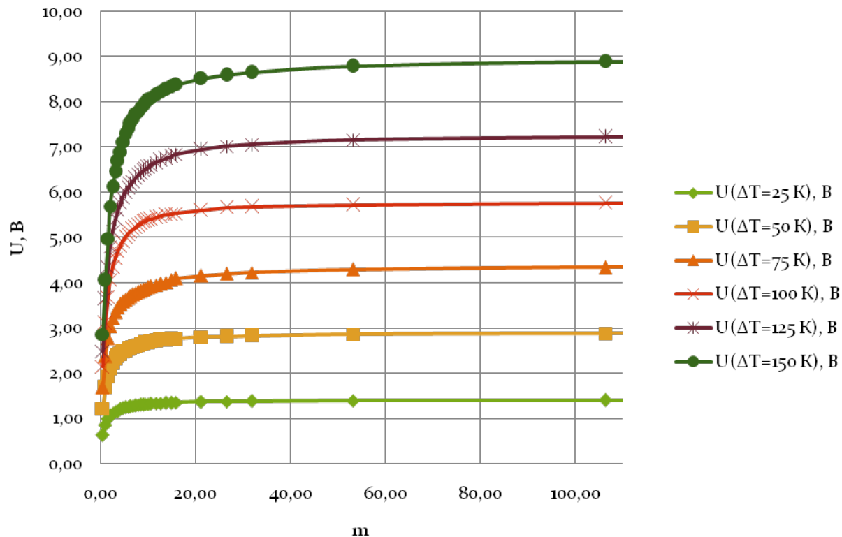
График зависимости U(\text{В}) от параметра m (см. (6)) для ТГМ-199-1,4-0,8
