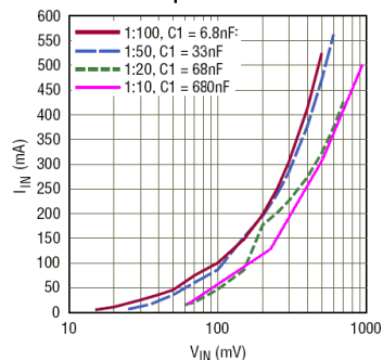
Типичная входной ток I_{IN} при Униполярном включении
