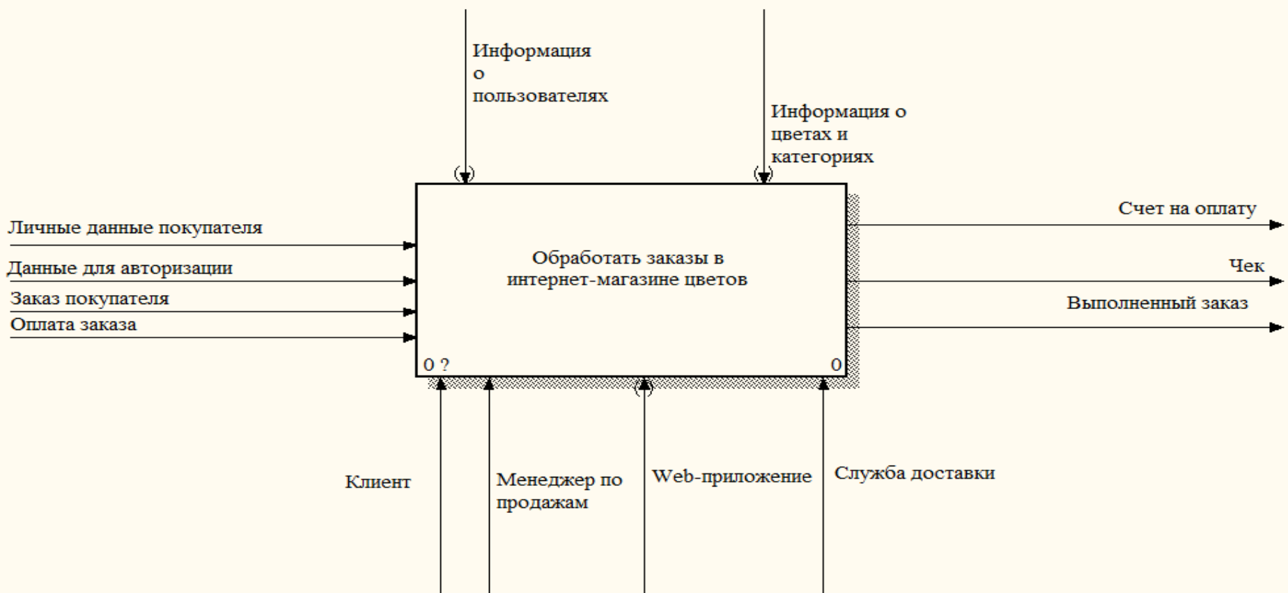
Рисунок 1.2 – Контекстная диаграмма.
